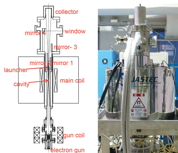
The cross-section and photo of a recently developed gyrotron. 左は最近開発した高性能ジャイロトロンの断面図及び写真。
