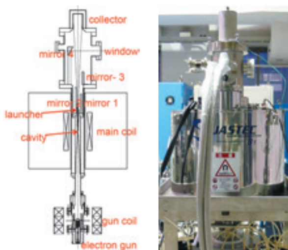
The cross-section and photo of a recently developed gyrotron. 左は最近開発した高性能ジャイロトロン断面図及び写真。
